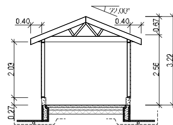
Snitt-tegning enkel garasje 3,20m bredde
