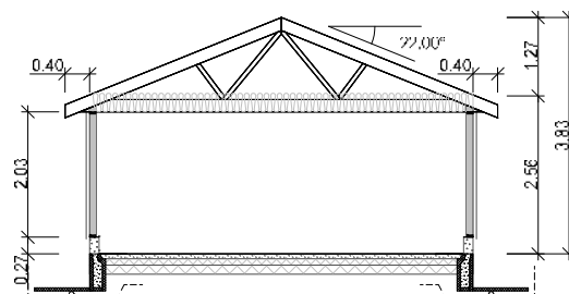
Snitt-tegning dobbel garasje 6,20m bredde uten loft.
