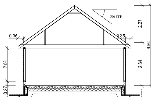
Snitt-tegning dobbel garasje 6,20m bredde med loft.
